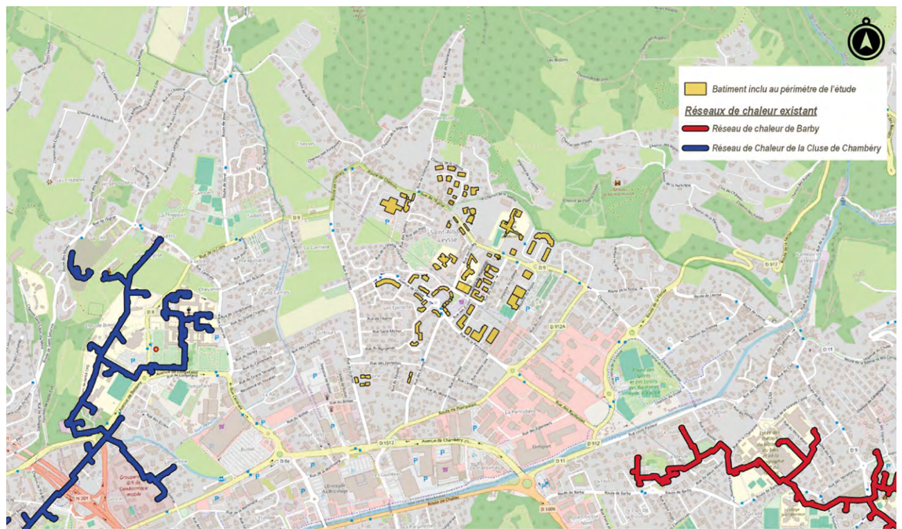
Étude de faisabilité chaufferie et réseau de chaleur. Sources : Open Street Map, Épos - Édité le 21/11/2025.
